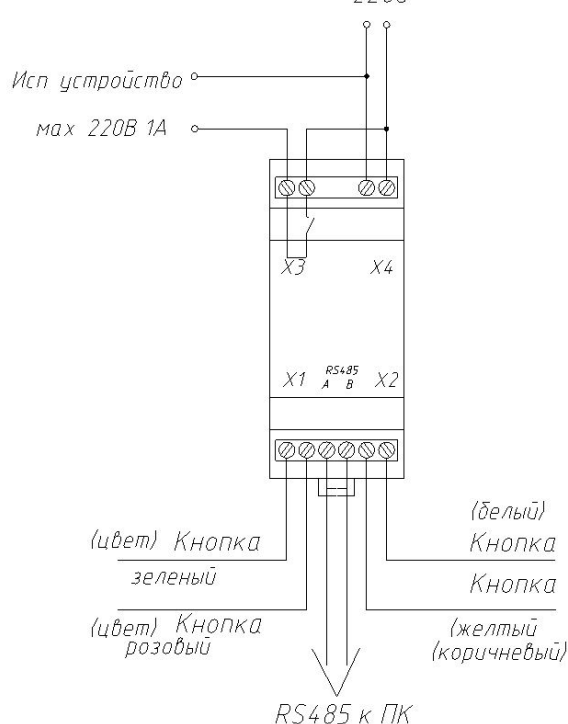
Схема подключения ~220В
